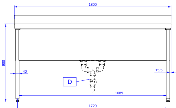
Bočna/o
